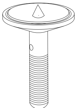
STEP A ( regolabile girevole con punta ) ( brass adjustable pin with tip )
